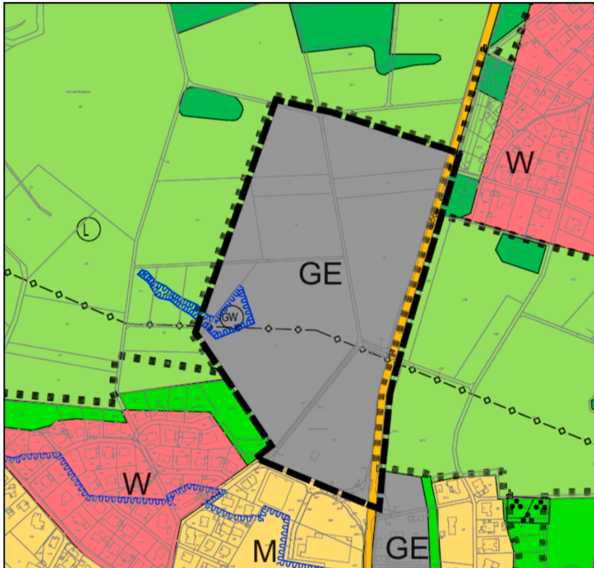
Abb. 7: Geplante Darstellung des Flächennutzungsplans, M: 1:5.000
